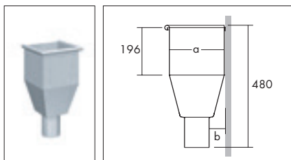
Sběrný kotlík hranatý, s kruhovým vývodem
