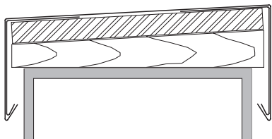
RHEINZINK - oplechování
