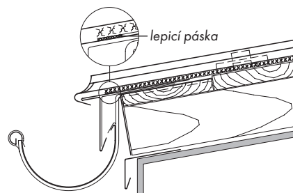
Ukončení okapnice, stojaté kulaté
