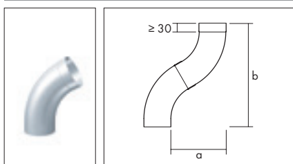
Koleno kruhové 60°
