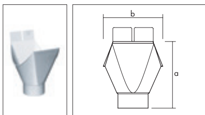
Kotlík závěsný půlkulový (tvar G)
