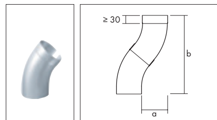
Koleno kruhové 40°
