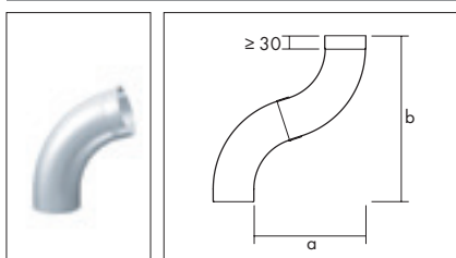
Koleno kruhové 72°
