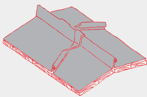
Nároží nebo hřeben jako dvojitá stojatá drážka
