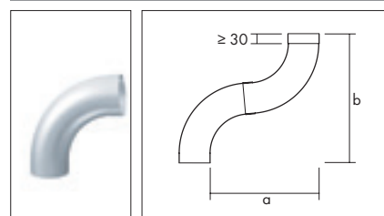
Koleno kruhové 85°
