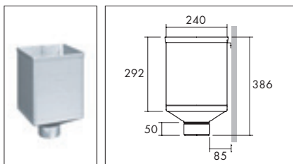
Sběrný kotlík QUADRO, s kruhovým vývodem
