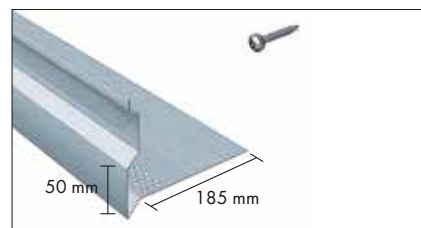
Vízszintes lábazati elem, csavarokkal
